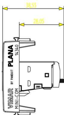
Vista ingombri
