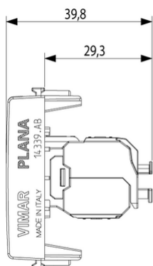
Vista ingombri
