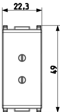
Vista ingombri
