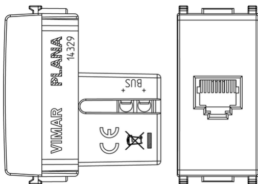
Vista ingombri
