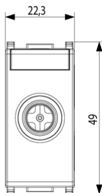
Vista ingombri
