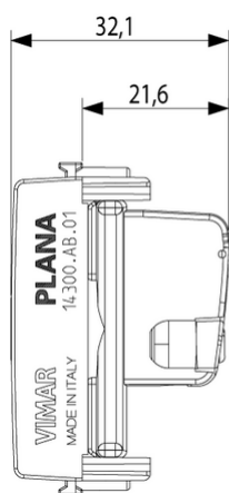
Vista ingombri
