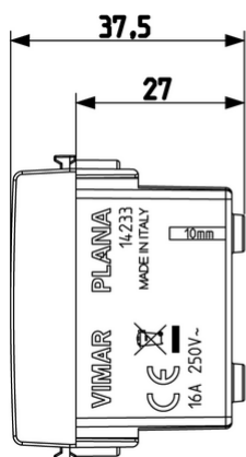
Vista ingombri
