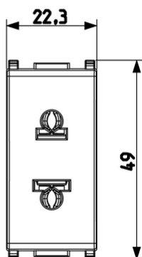
Vista ingombri
