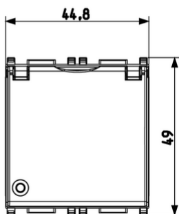
Vista ingombri
