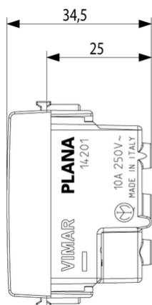
Vista ingombri
