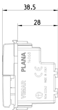
Vista ingombri
