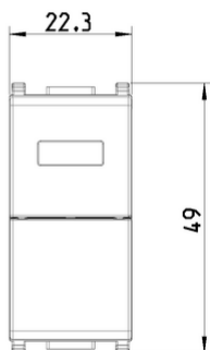
Vista ingombri
