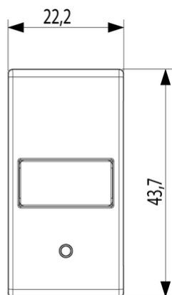
Vista ingombri
