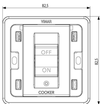
Vista ingombri
