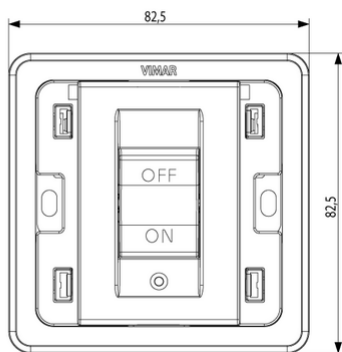
Vista ingombri
