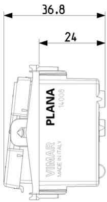
Vista ingombri
