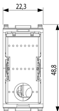
Vista ingombri
