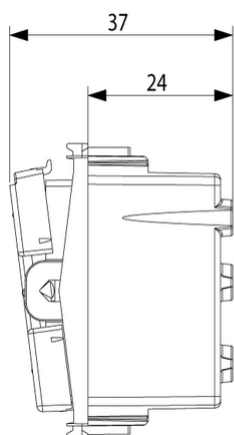
Vista ingombri
