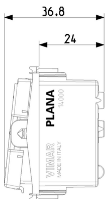
Vista ingombri
