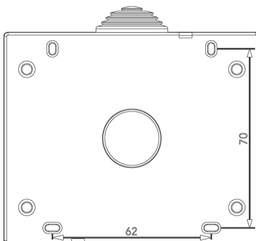
Vista posteriore
