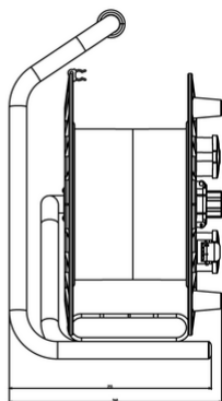
Vista ingombri
