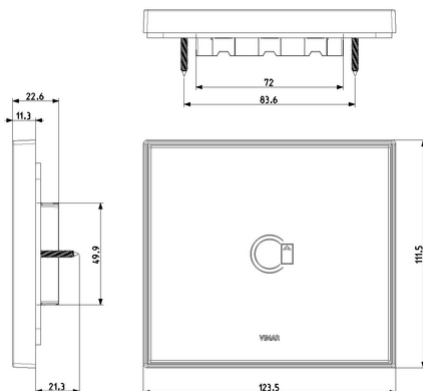
Vista ingombri
