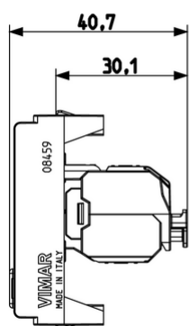
Vista ingombri
