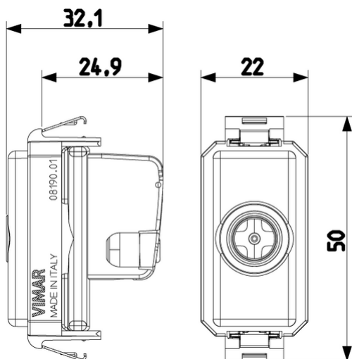
Vista ingombri
