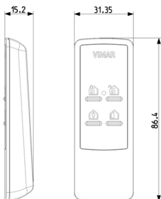
Vista ingombri
