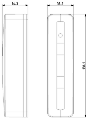
Vista ingombri
