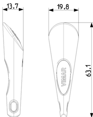
Vista ingombri
