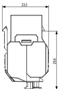
Vista ingombri
