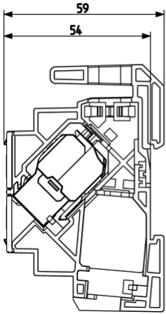
Vista ingombri
