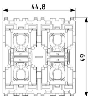
Vista ingombri
