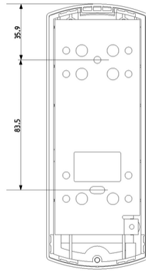
Vista posteriore
