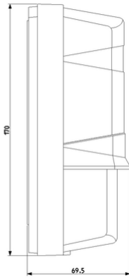
Vista ingombri
