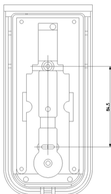
Vista posteriore
