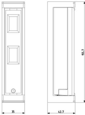
Vista ingombri
