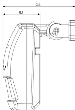
Vista ingombri
