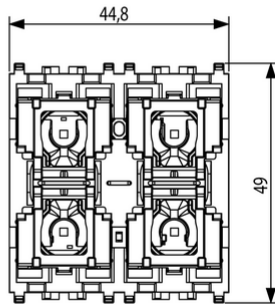
Vista ingombri
