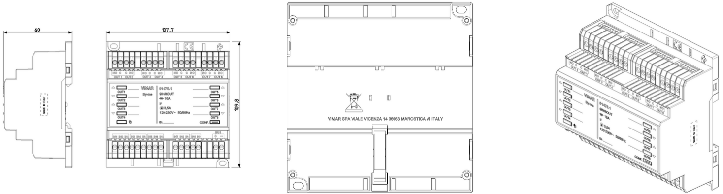
Vista ingombri
