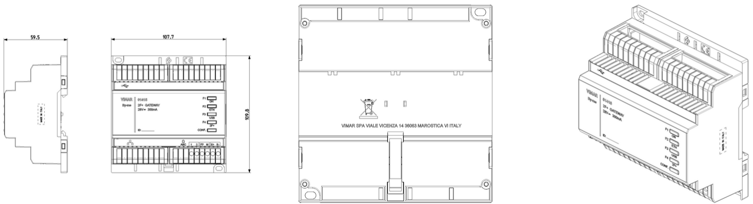
Vista ingombri
