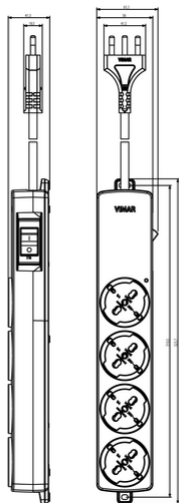
Vista ingombri
