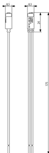
Vista ingombri
