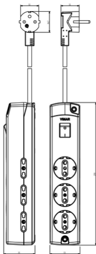
Vista ingombri
