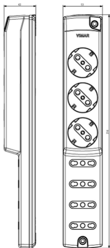
Vista ingombri
