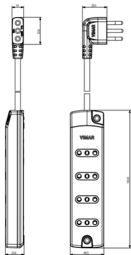
Vista ingombri
