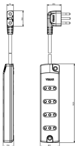
Vista ingombri
