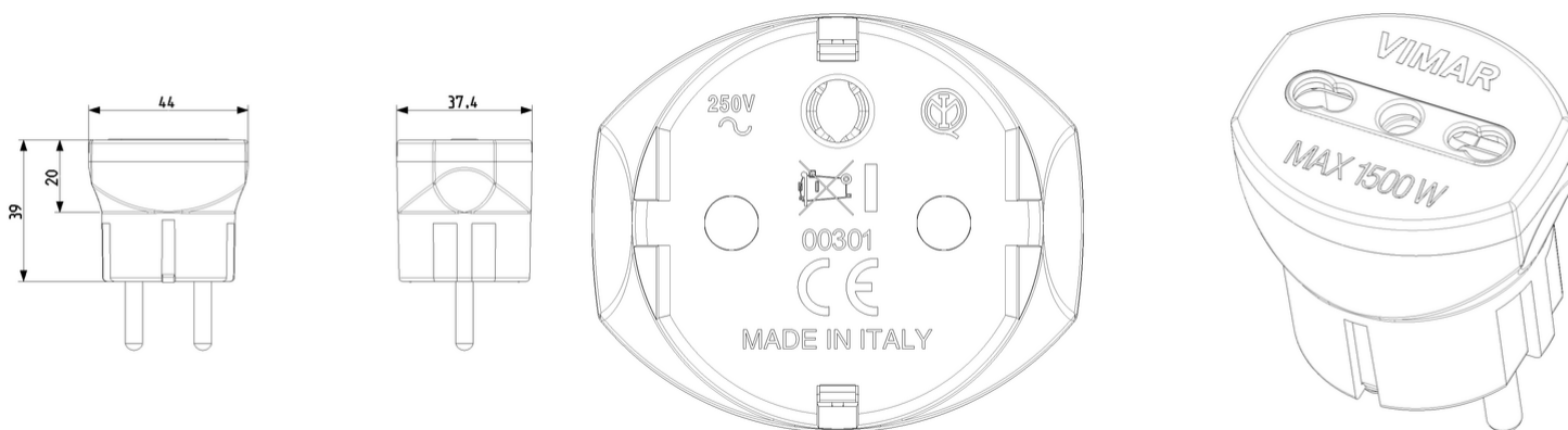
Vista ingombri
