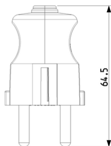
Vista ingombri
