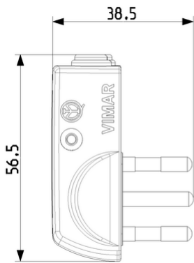
Vista ingombri
