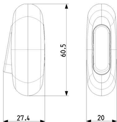
Vista ingombri
