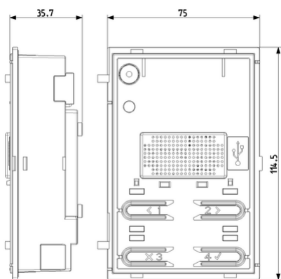
Vista ingombri
