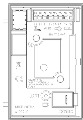
Vista posteriore
