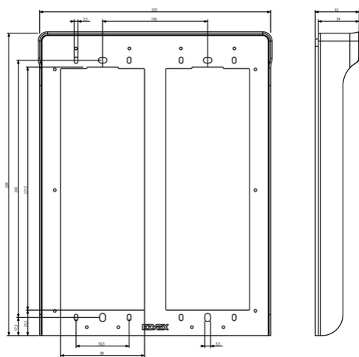
Vista ingombri
