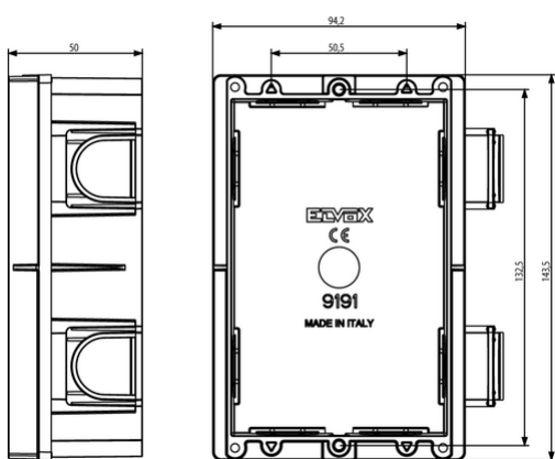
Vista ingombri
