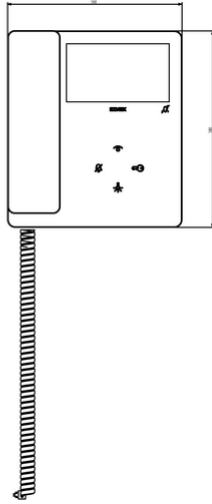
Vista ingombri
