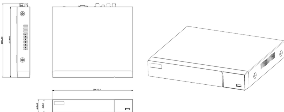
Vista ingombri
