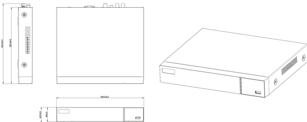
Vista ingombri
