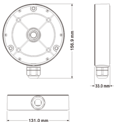
Vista ingombri
